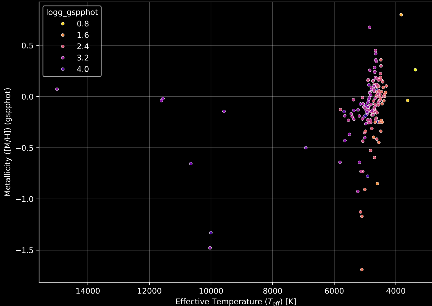
APOGEE DR17 Field: [000-08] Stellar Population Parameters (n= 175)
